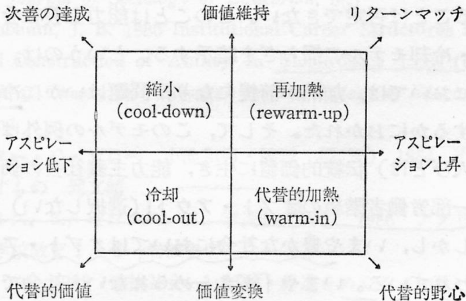
図4-2 失敗への適応類型
